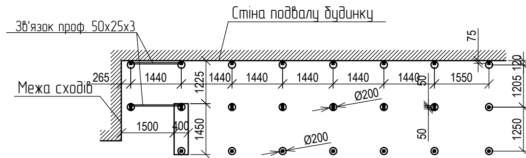
План фундаментів та стійок
